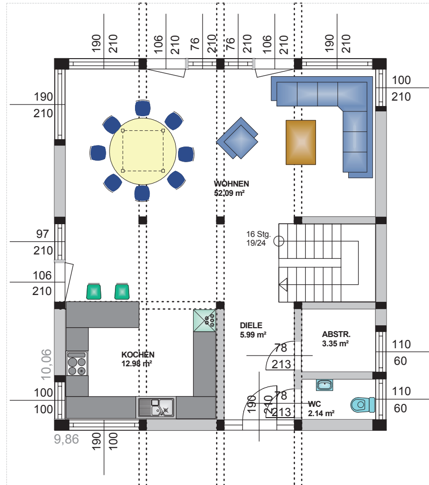
ERDGESCHOSS
